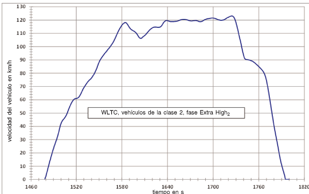
Figura A1/6 WLTC, vehículos de la clase 2, fase Extra High 2
