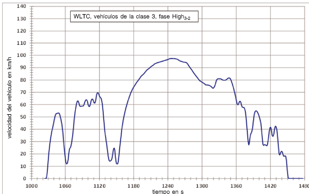
Figura A1/11 WLTC, vehículos de la clase 3, fase High 3-2
