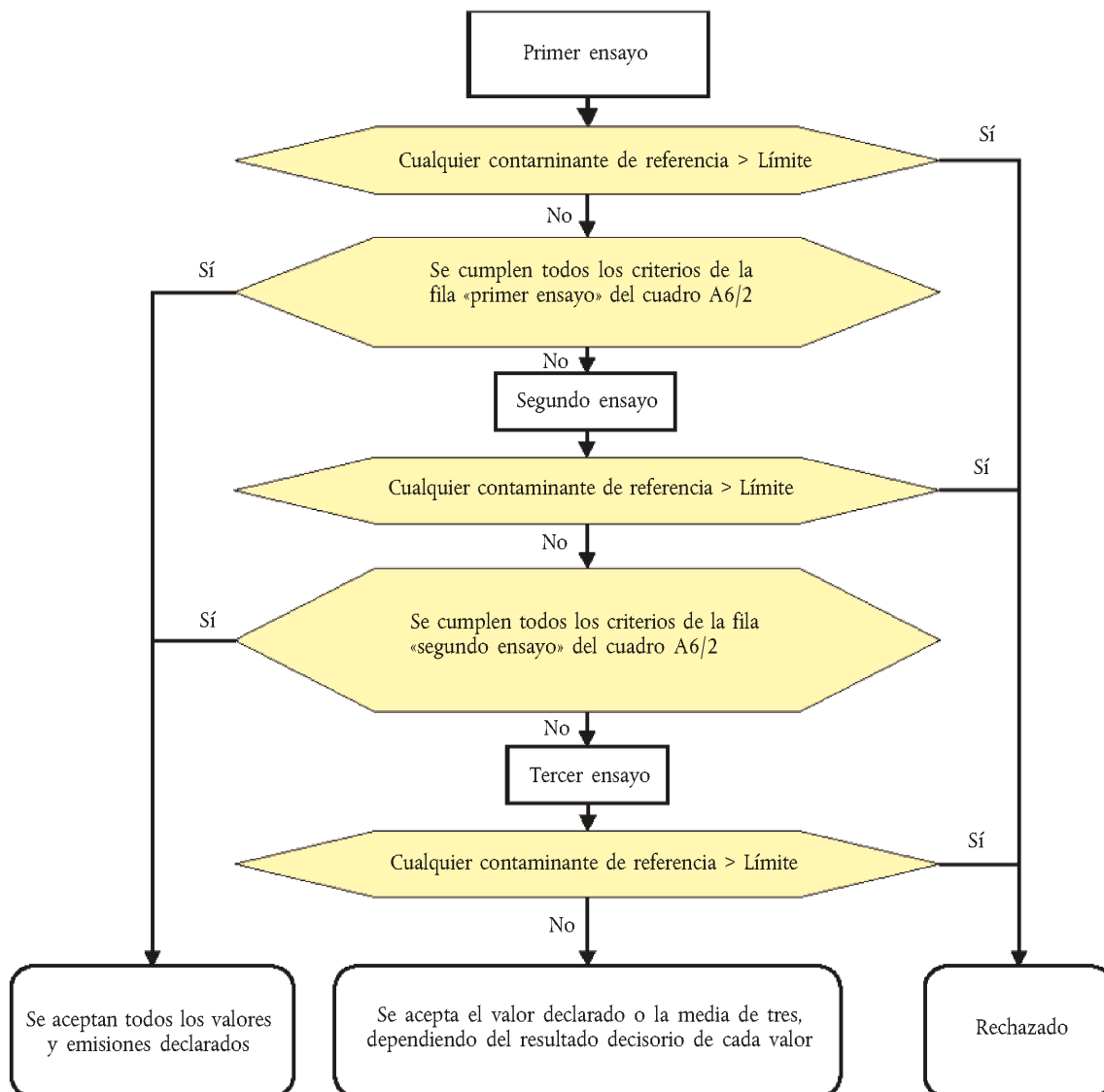
Figura A6/1 Organigrama del número de ensayos de tipo 1
