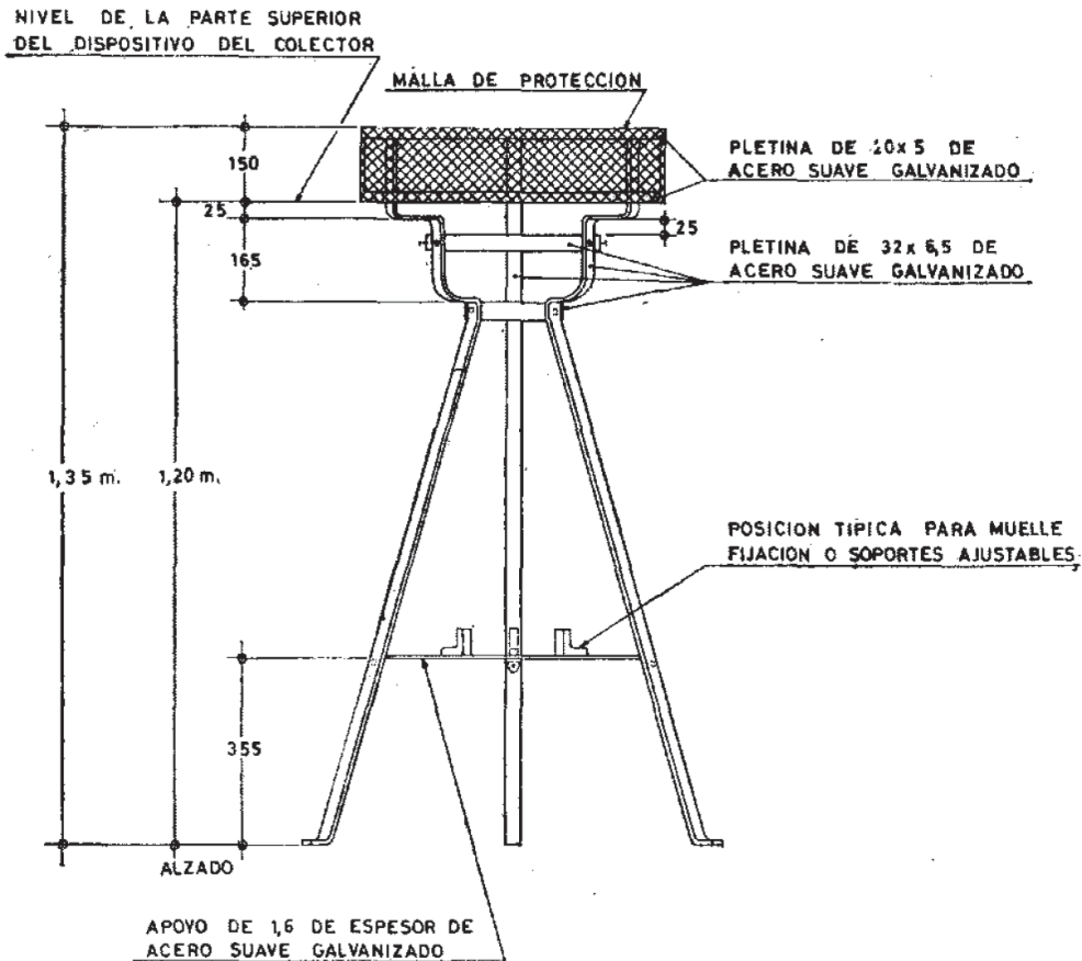
Figura 9. Soporte con rejilla protectora
