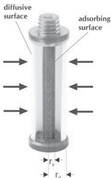
Figura 20. Esquema del fundamento de la difusión radial. (Fuente: Manual Radiello).
