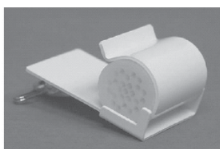
Figura 14. Captador pasivo Ogawa. (Fuente: Manual Radiello).
