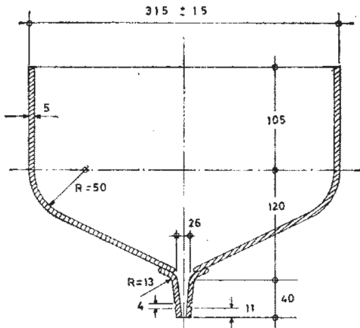
Figura 10. Depósito colector
