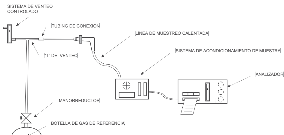
Figura 6. Analizador de gases de combustión mediante células electroquímicas. Configuración de calibración/verificación.
