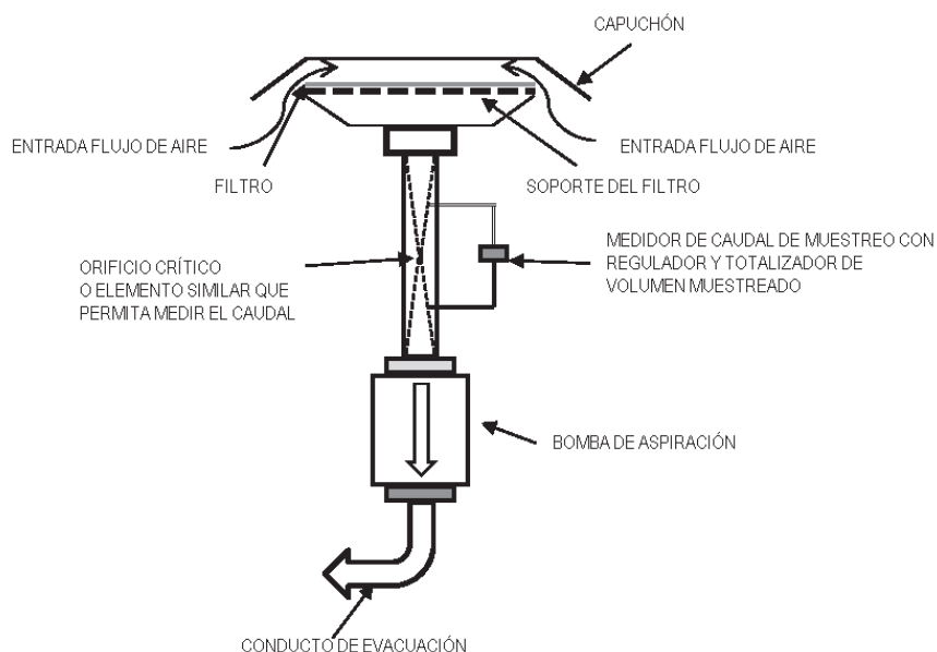
Figura 7. Esquema de funcionamiento de un captador de alto volumen
