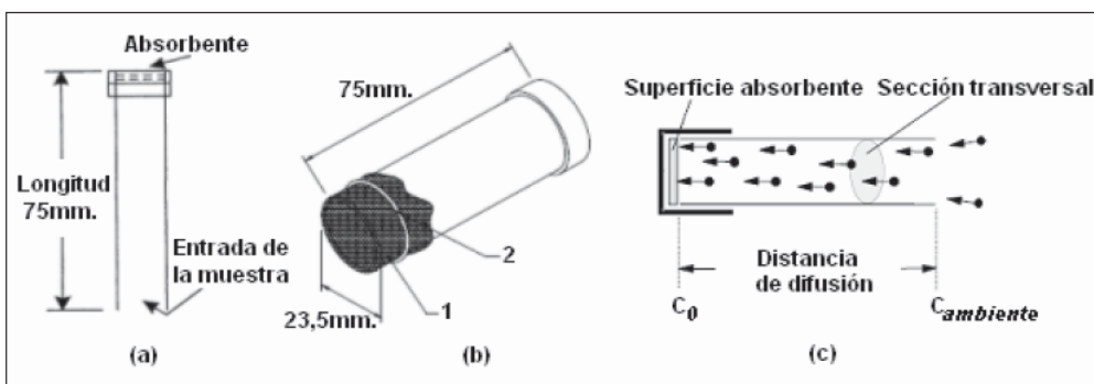
Figura 16.(a) y (b) Tubo Palmes. (c) Esquema de funcionamiento.
