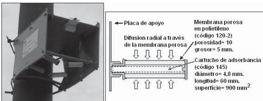
Figura 22. Detalle de colocación y fundamento de la difusión radial. (Fuente: Manual Radiello.)
