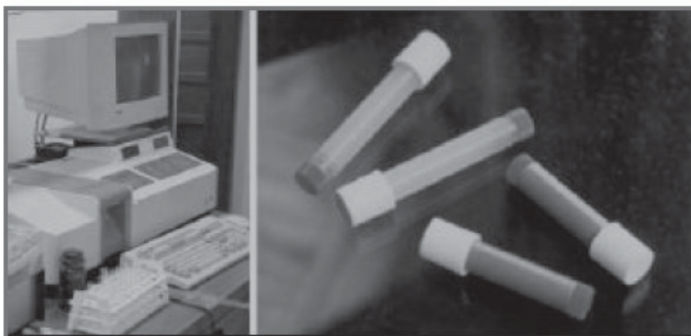
Figura 17. Espectrofotómetro utilizado para el análisis de tubos y ejemplos de tubos captadores (NO 2 los dos de arriba –blancos- y O 3 los dos de abajo –azules-). (Fuente: Manual Radiello).
