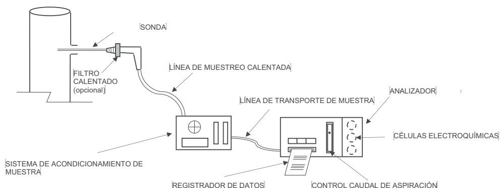
Figura 5. Analizador de gases de combustión mediante células electroquímicas. Configuración de medida.
