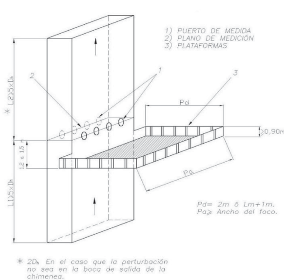
Figura 3. Detalle de la ubicación de los orificios de muestreo y dimensiones de la plataforma en conductos rectangulares.
