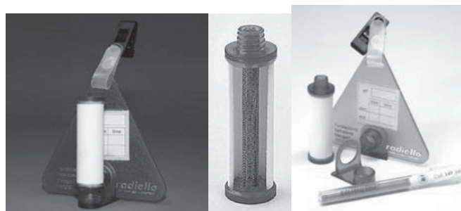
Figura 19. Captador passivo Radiello montado. Cartucho o filtro impregnado. Captador desensamblado. (Fuente: Manual Radiello).
