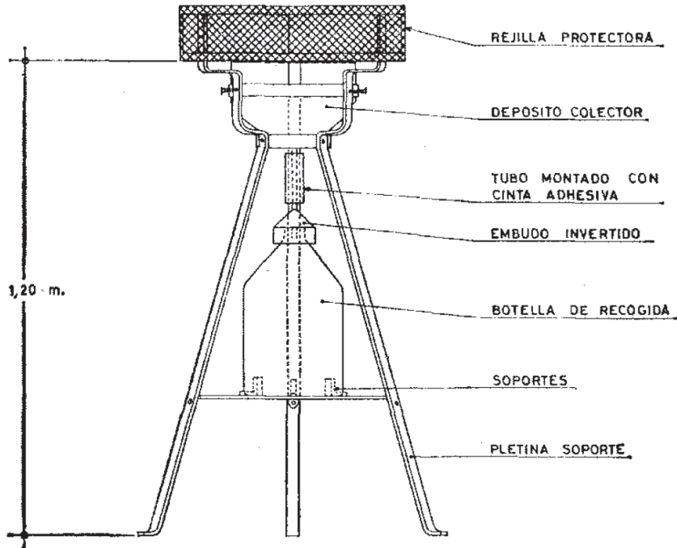
Figura 8. Conjunto del equipo colector
